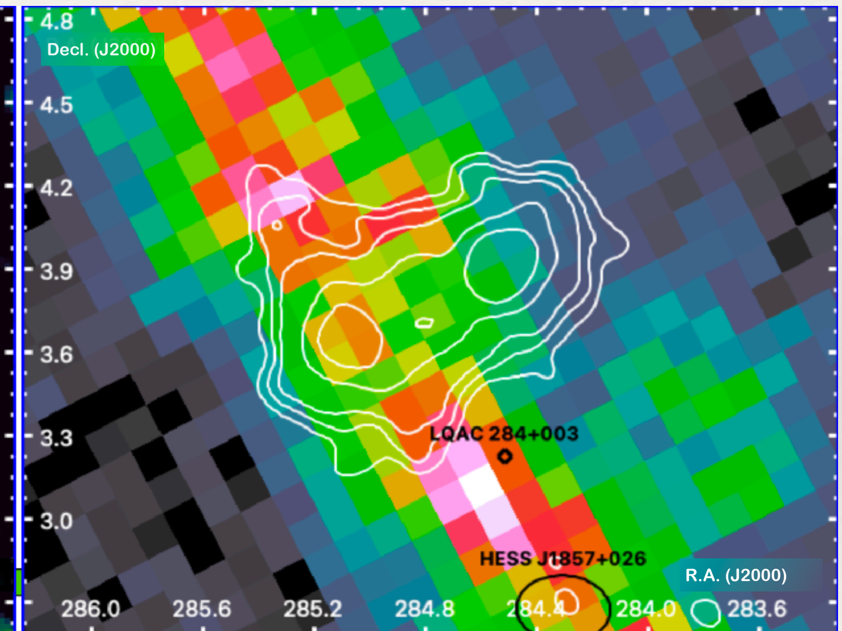
1LHAASO J1858+0330 (4FGL J1858.0+0354 & 4FGL J1900.4+0339)
