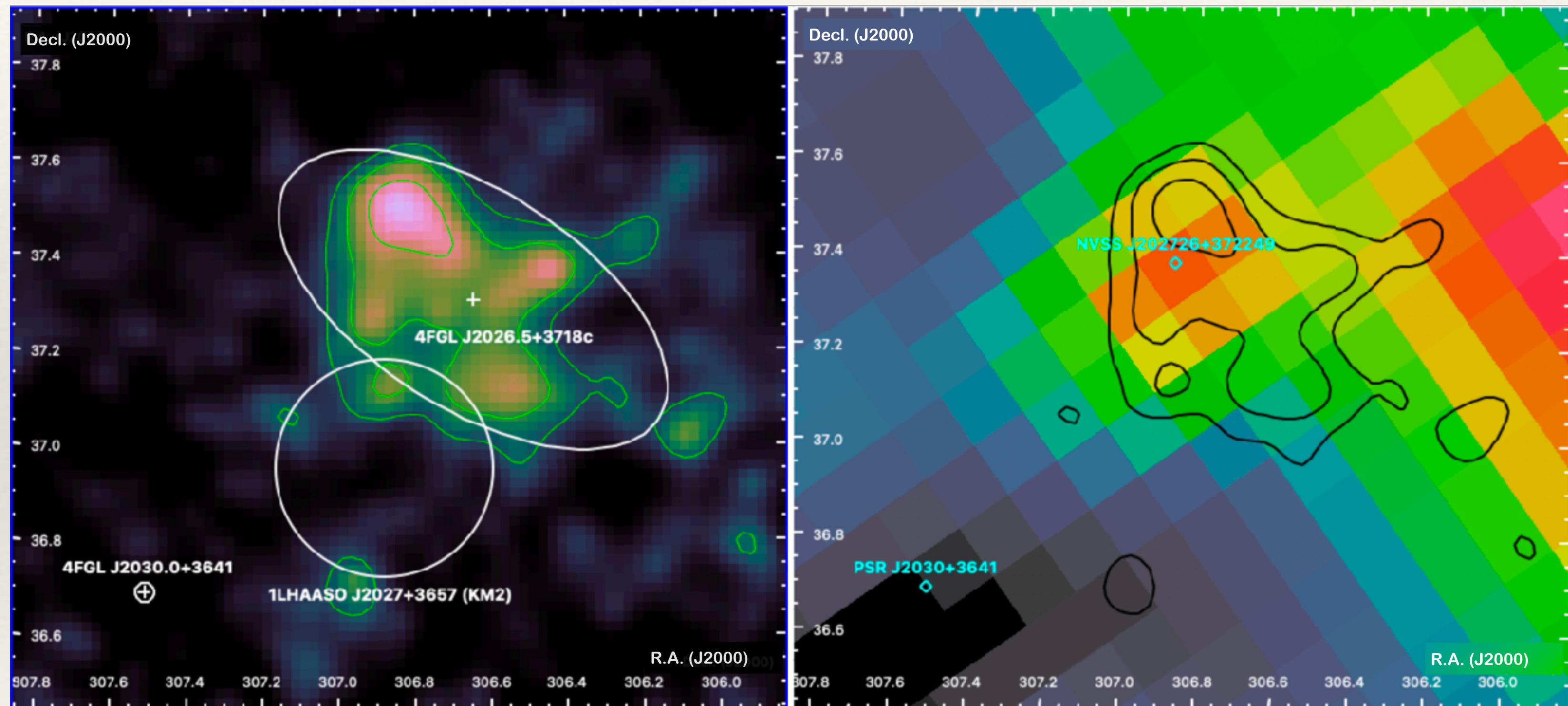
1LHAASO J2027+3657 (4FGL J2026.5+3718c)
