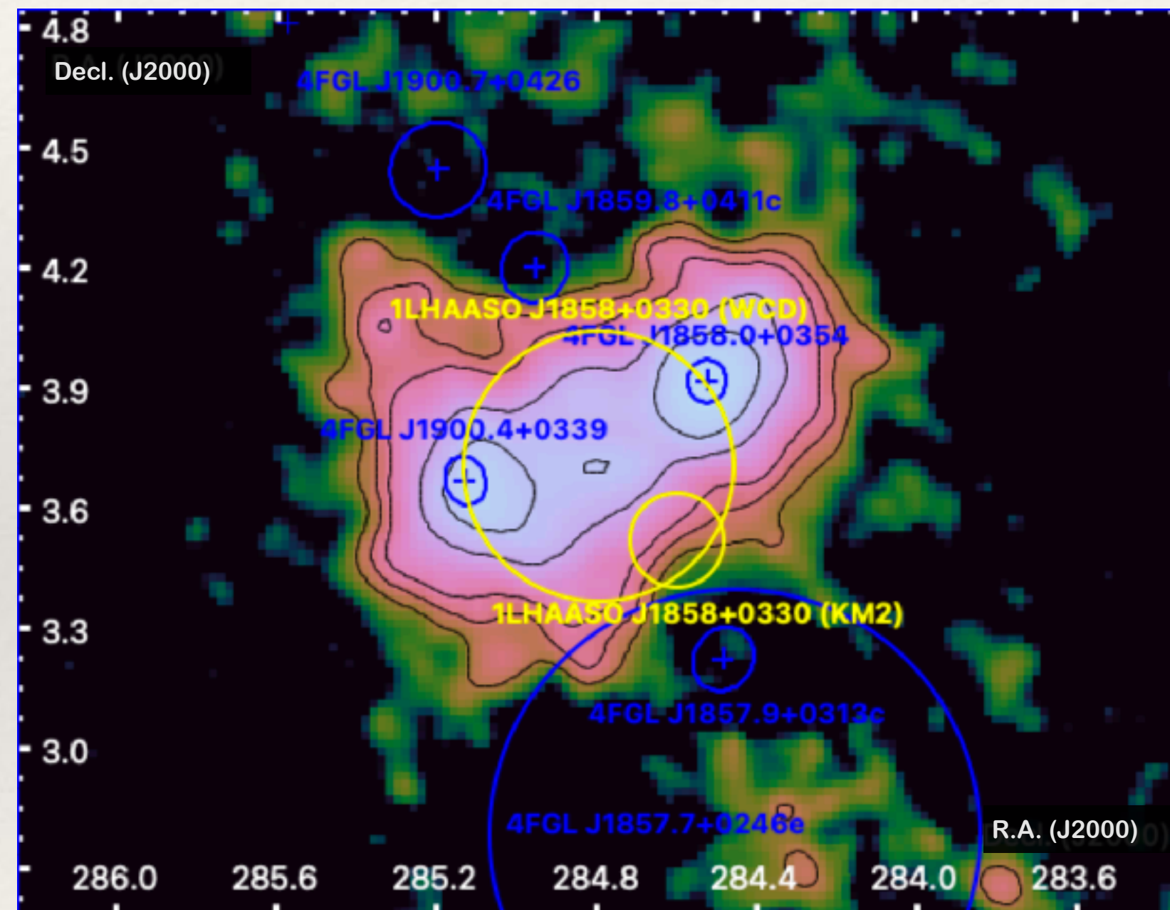
1LHAASO J1858+0330 (4FGL J1858.0+0354 & 4FGL J1900.4+0339)
